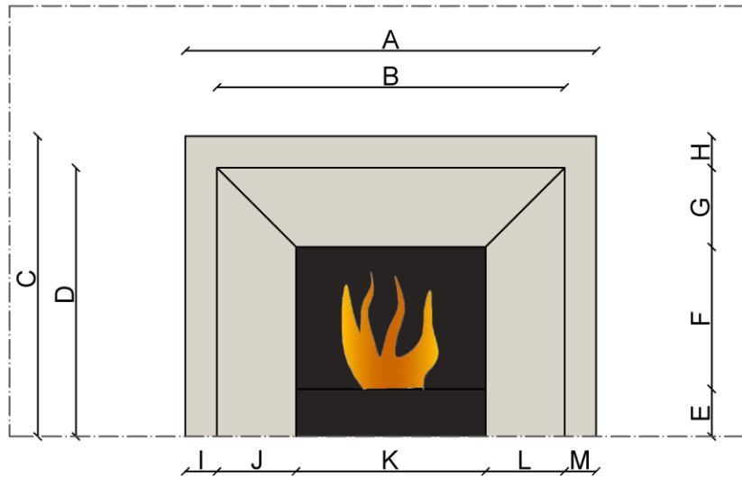
Prospetto frontale
