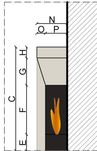
Sezione laterale
